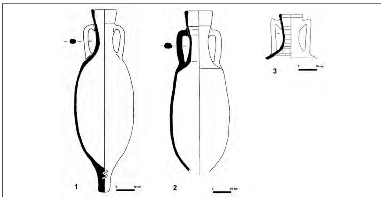
FIGURA 19. 1) Àmfora Pascual 1 del període 15 aC - 20 dC; 2) àmfora Pascual 1 del període 20 dC - 75 dC; 3) àmfora Dressel 2-3 del període 20 dC - 75 dC (Carbonell et al. , 1989).
