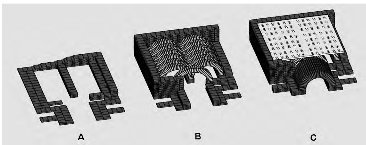
FIGURA 18. A) Esquema constructiu del forn 1, amb la disposició dels tovots sesquipedals rectangulars; B) restitució dels arcs de maons cuits, pedales , basada en els inicis d'aquests; C) restitució de la graella i de la volta del praefurnium . Dibuix de l'autor.
