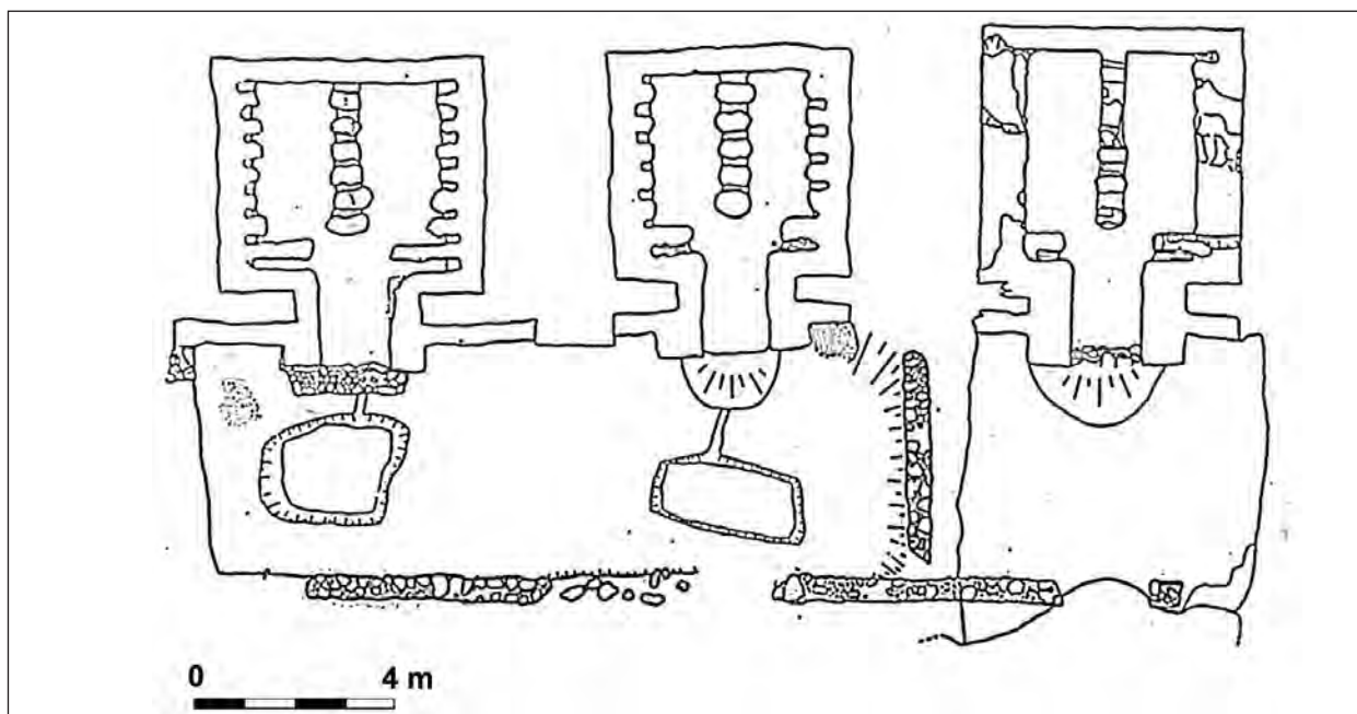
FIGURA 17. Planta del forn 1 (dreta), forn 2 (centre) i forn 3 (esquerra). Davant dels forns 2 i 3 s'han documentat unes cubetes amb canal que probablement drenaven l'aigua pluvial durant la construcció amb tovots dels forns, i que van ser reblertes un cop construïts. Planimetria: Servei d'Arqueologia i Paleontologia.
