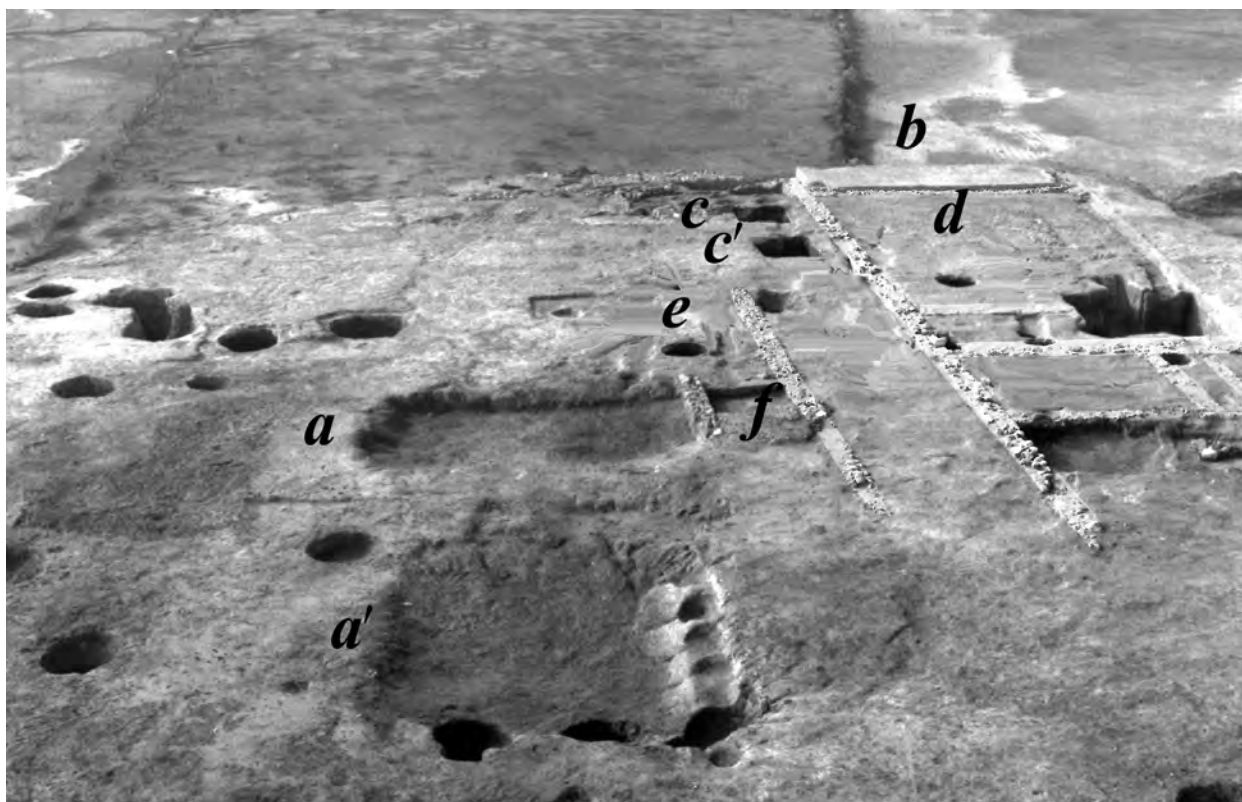
FIGURA 15. Fotografia aèria del sector de l'edifici. a i a' ) Basses de decantació d'argiles; b ) lacus ; c i c' ) fosses dels contrapesos de les premses; d ) àmbit de les premses; e ) pou d'aigua; f ) dipòsit. S'hi observen nombroses sitges i estructures de fases precedents. Fotografia: Institut Cartogràfic i Geològic de Catalunya.
