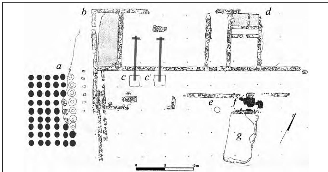
FIGURA 13. Planta de l'edifici. a) Magatzem de dolia (part excavada i restitució hipotètica); b) lacus ; c i c') fosses dels contrapesos de les premses ( arcae lapidum ) i restitució hipotètica de les bigues; d) possible calcatorium ; e) pou d'aigua; f) dipòsit; g) bassa oest de decantació d'argiles. Restitució de les premses basada en Martín Oliveras i Bayés, 2009, p. 234, fig. 18. Planimetria: Servei d'Arqueologia i Paleontologia.
