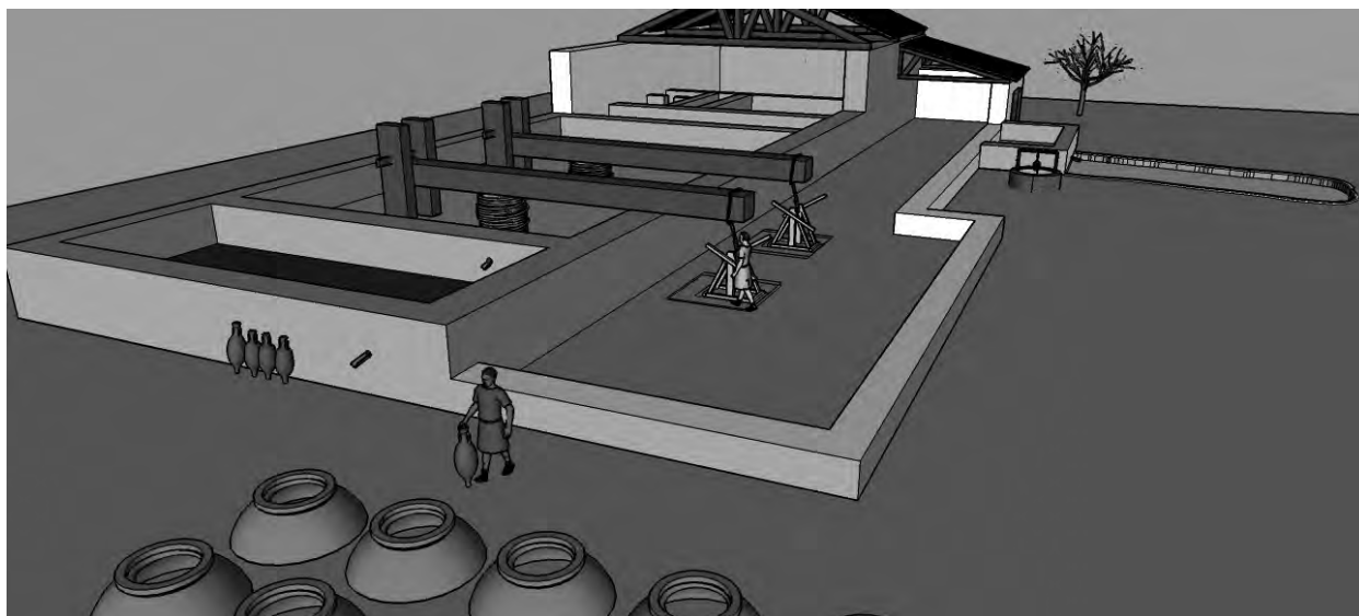
FIGURA 14. Esbós interpretatiu del complex de producció de vi (dibuix de l'autor): premses, lacus i magatzem de dolia . A la dreta, pou d'aigua i bassa oest de decantació d'argiles. Tipologia de premses basada en Martín Oliveras i Bayés, 2009.
